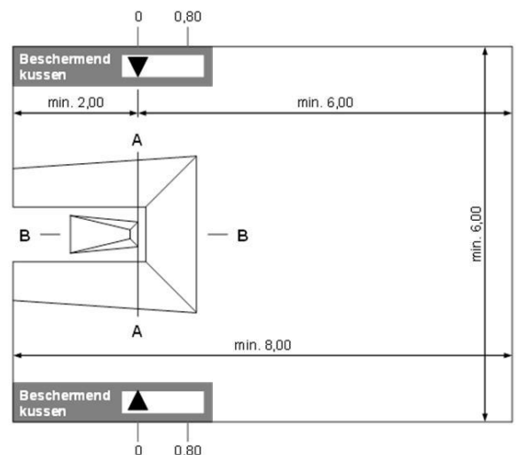
Bovenaanzicht (alle afmetingen in m)
