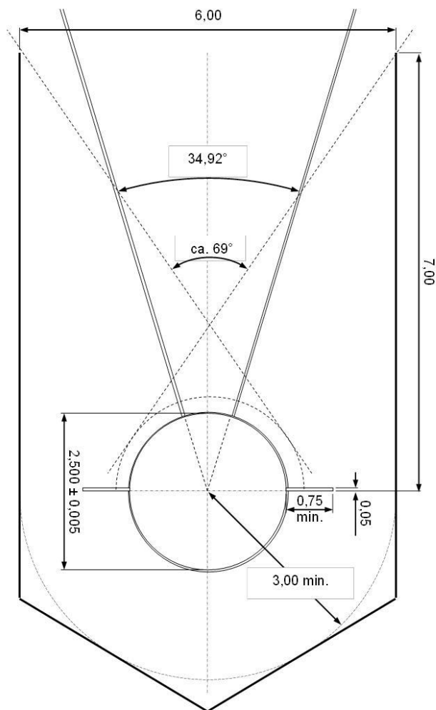
Fig. 190 Plattegrond van een discuskooi (alle afmetingen in m)
