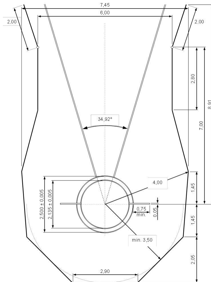
Fig. 192b Kooi voor discuswerpen en kogelslingeren Panelen in stand discuswerpen (alle afmetingen in m)
